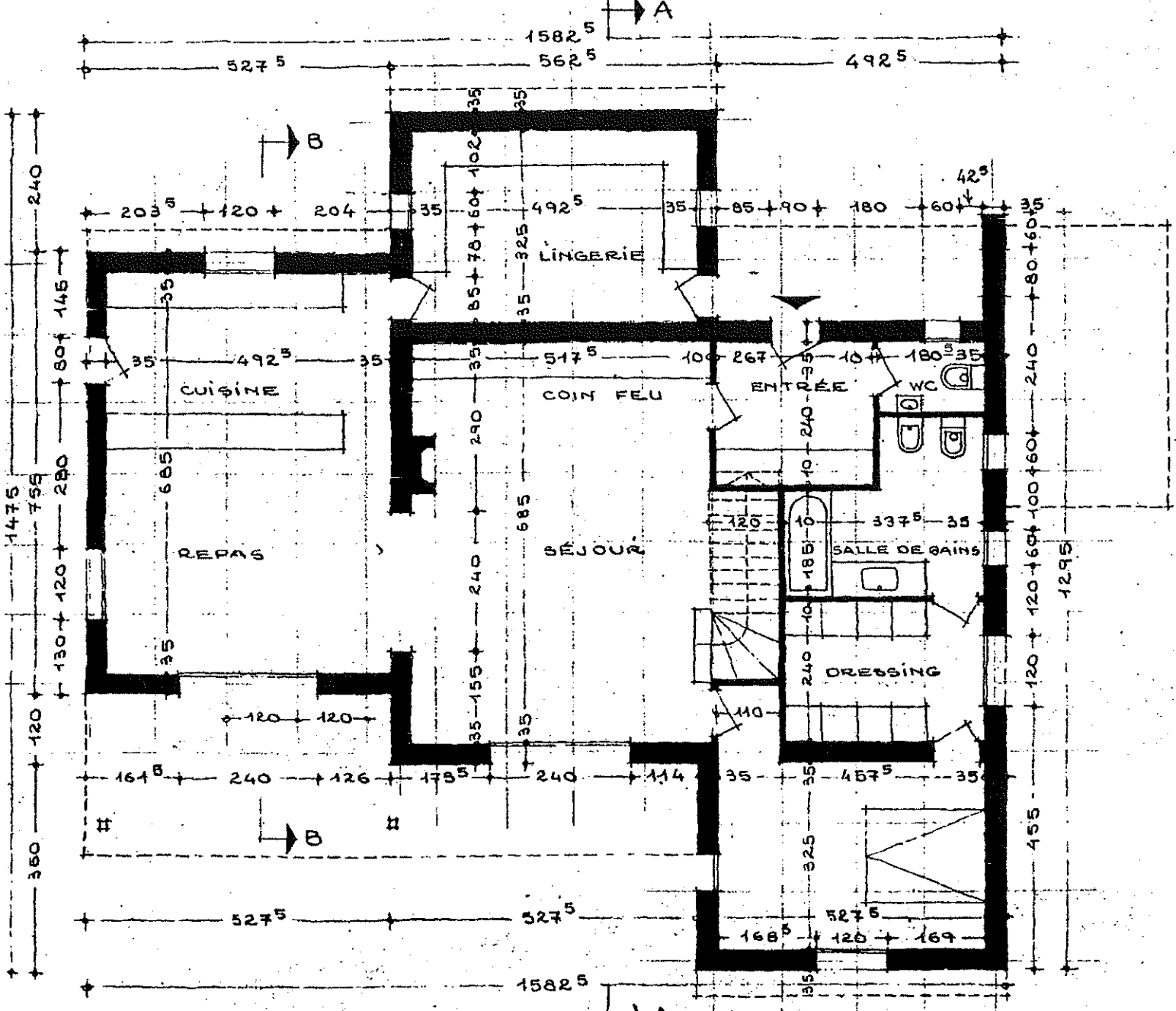
REZ. DE CHAUSSEE 1:100
