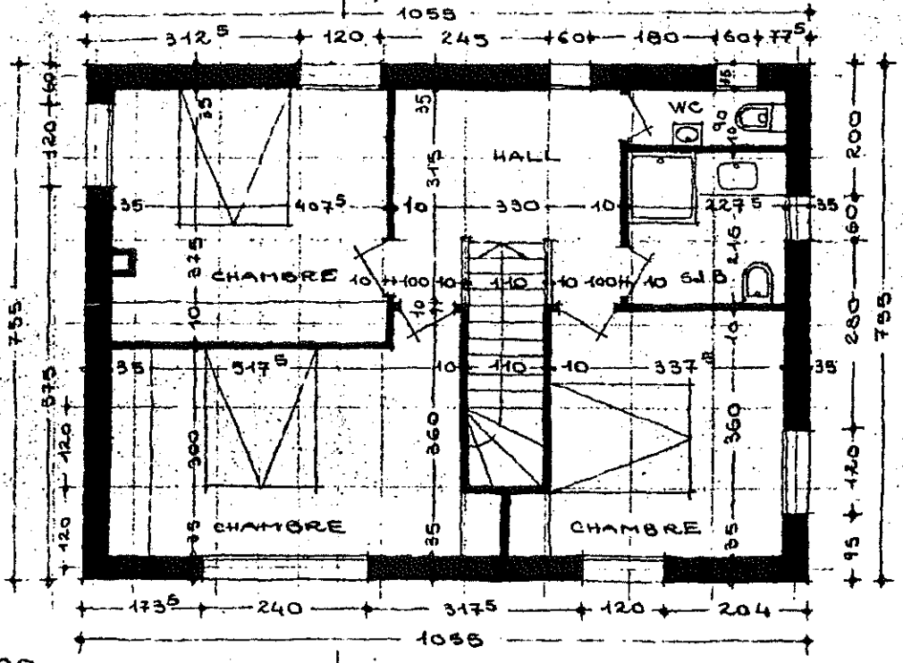
REZ. DE CHAUSSEE 1:100
